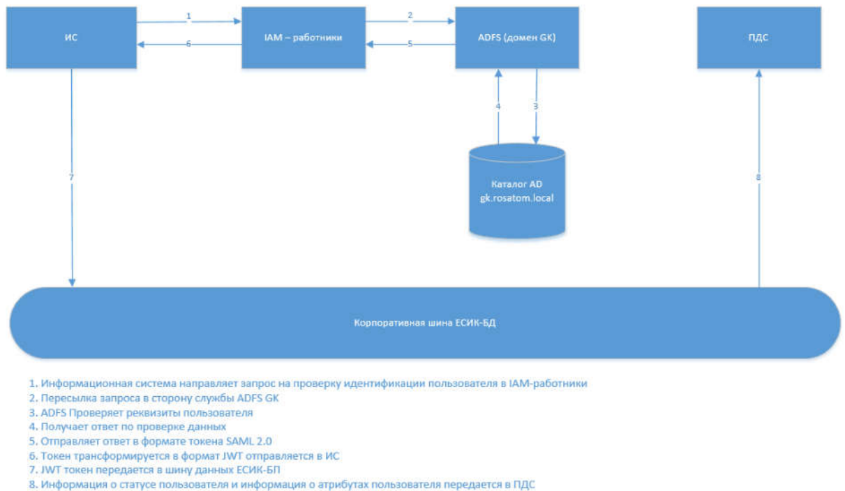
Рис. 3 схема описания передачи идентификационного токена через IAM
